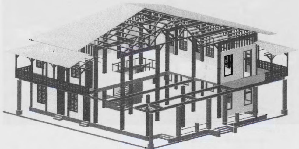
Abb. 9: Montagebau Haus Nr. 2, Gerichtsgebäude in Dar-es-Salaam Nachweis: Aufnahme des Autors.
