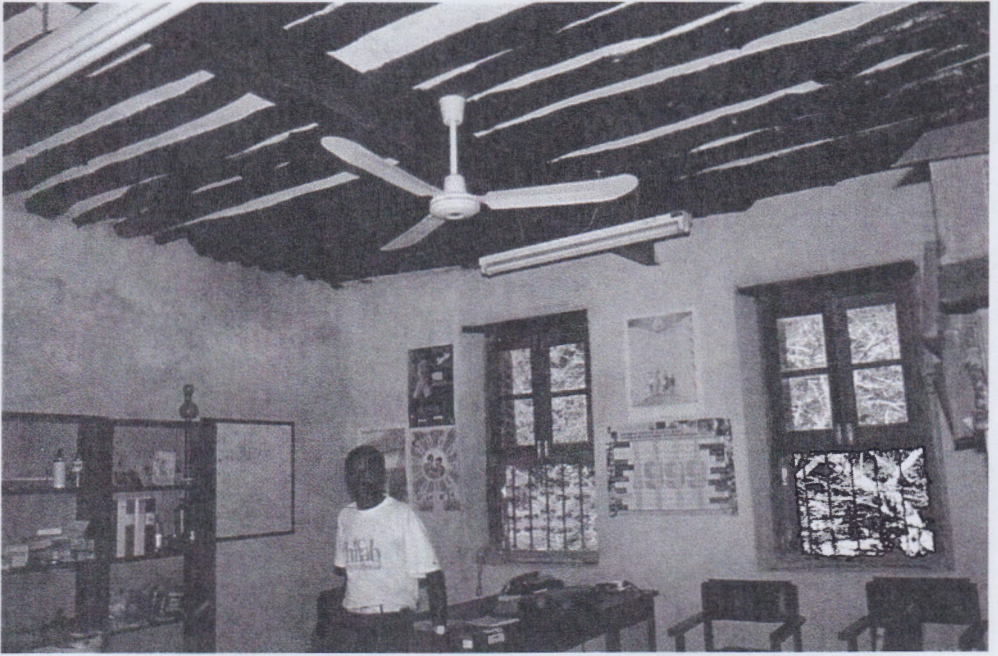
Abb. 6: Eine Wand wurde zum Abfangen der Deckenlast durch einen Stahlträger ersetzt. Nachweis: Aufnahme des Autors.
