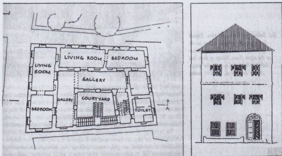
Abb. 4: Grundriß und Ansicht eines arabischen Hauses Nachweis: Abdul SHERIFF, The History and Conservation of Zanzibar Stone Town, London 1992.
